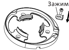
Рисунок 2-5 Установка зажима
