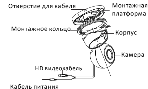
Рисунок 1-2 Камера II типа
