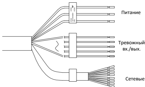
Рисунок 2-3 Обзор кабелей
