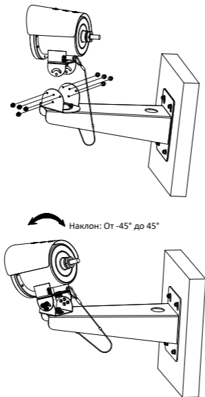
Рисунок 3-5 Закрепление камеры на настенном кронштейне
