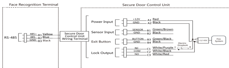
Рисунок 4-4 Подключение устройства
